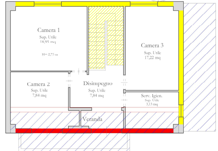
Piano Primo Scala 1:100
