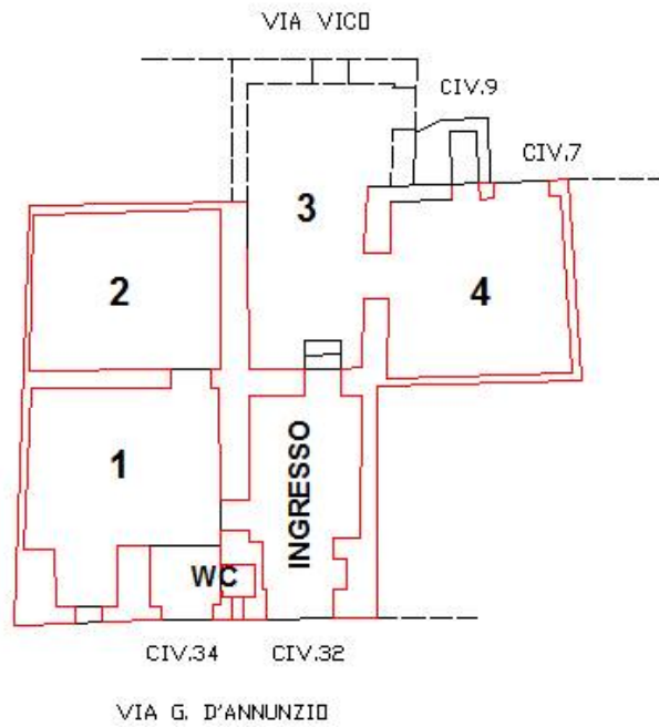
Planimetria con localizzazione ambienti
