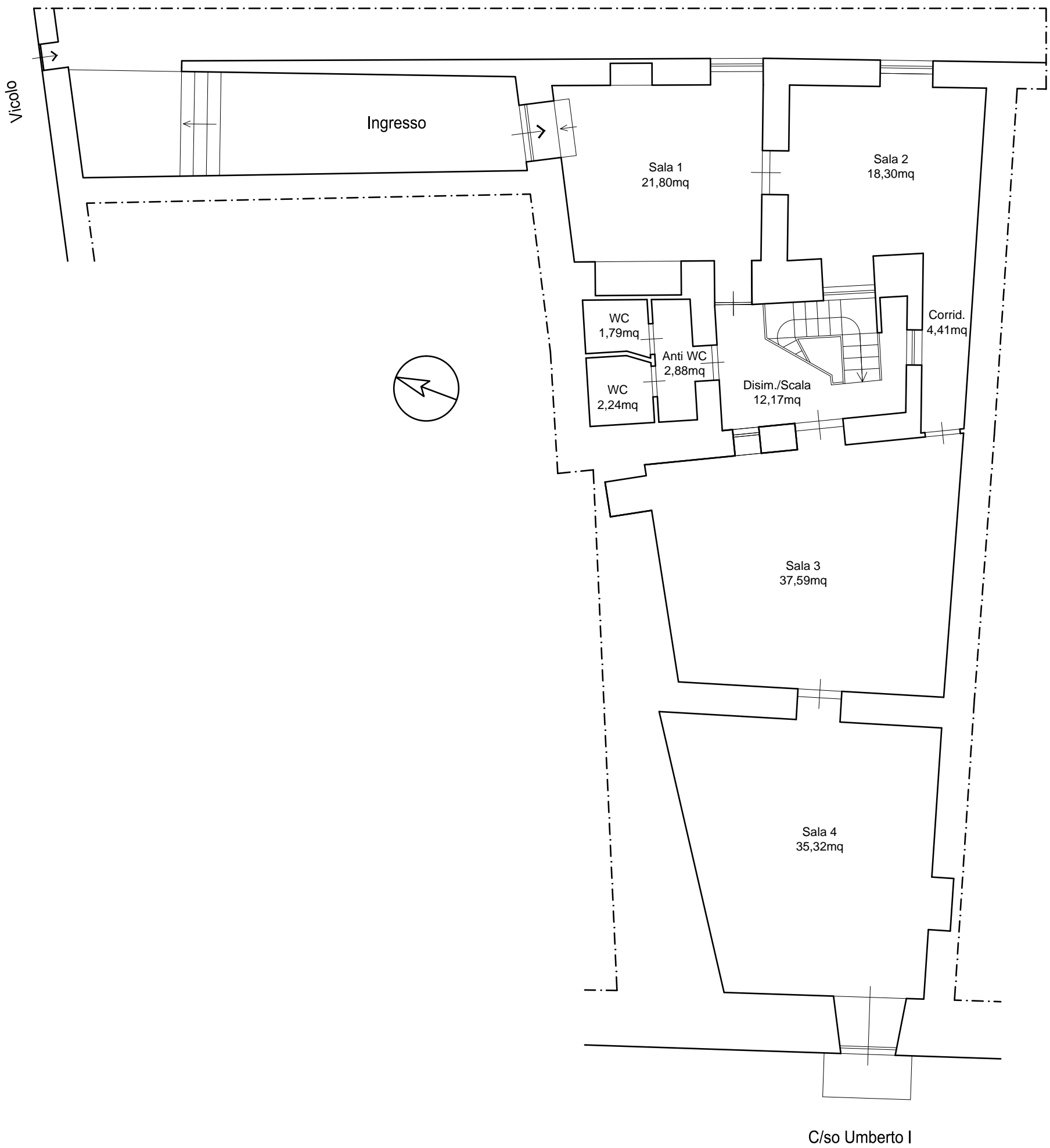
Pianta immobile Scala 1:100
