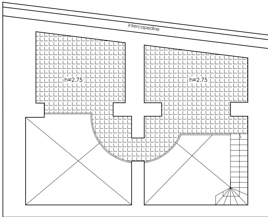
Piano Primo
