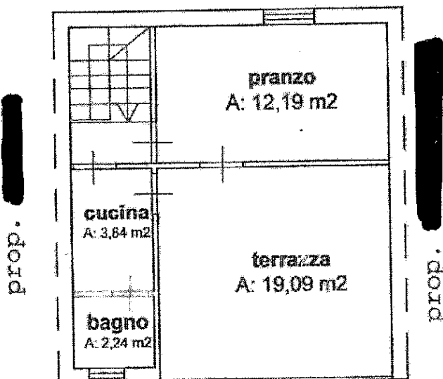
Corso Umberto I PIANTA PIANO TERZO h=2,55 superficie lorda A: 27,93 m 2
