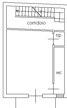
PIANTA PIANO SECONDO H= cm 300
