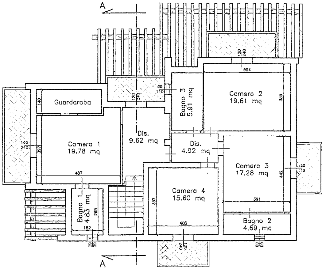
Pianta piano primo 1:100
