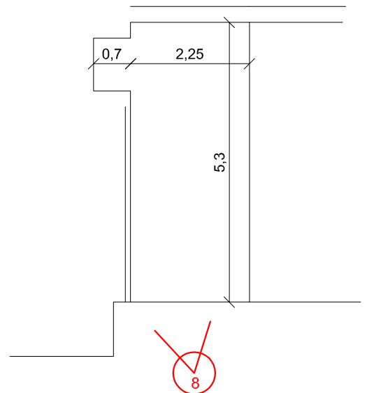
PIANTA POSTO AUTO COPERTO
