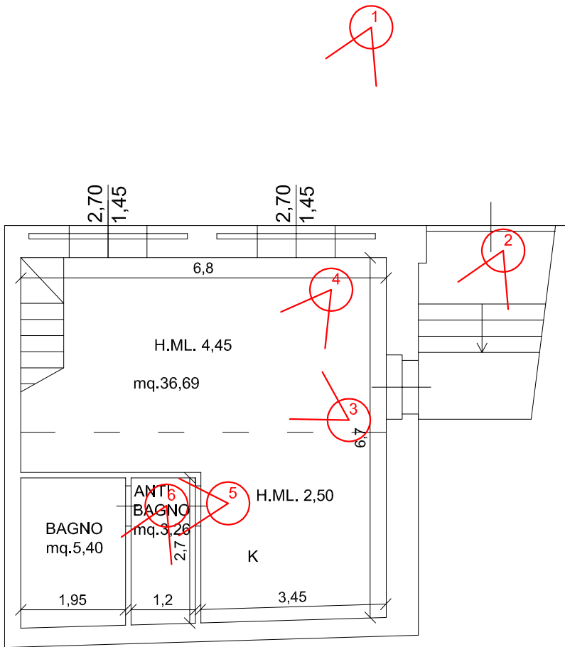
PIANTA CIVILE ABITAZIONE
