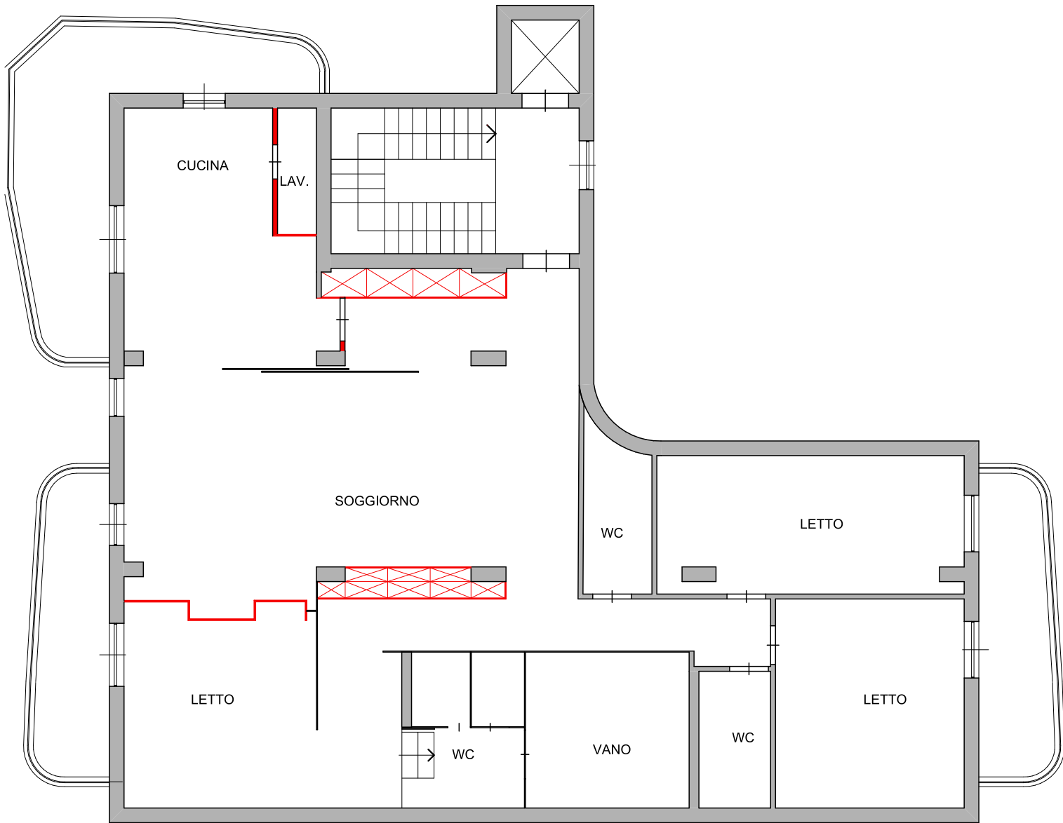
PIANTA DI PROGETTO scala 1:100
