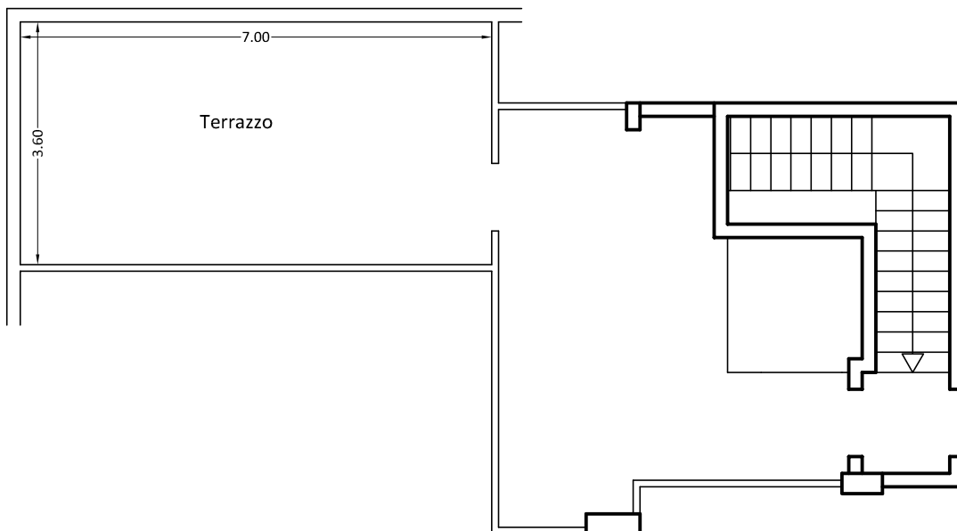
PLANIMETRIA TERRAZZO
