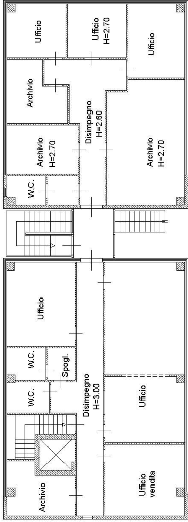
PIANO PRIMO
