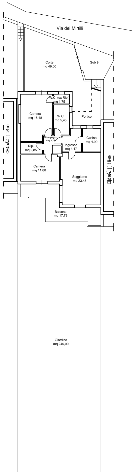
PIANTA STATO DI FATTO scala 1:200
